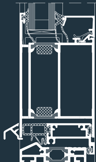
Schüco ADS 75.SI HD, målestoksforhold 1:2 Schüco Door ADS 75.SI HD, Scale 1:2
